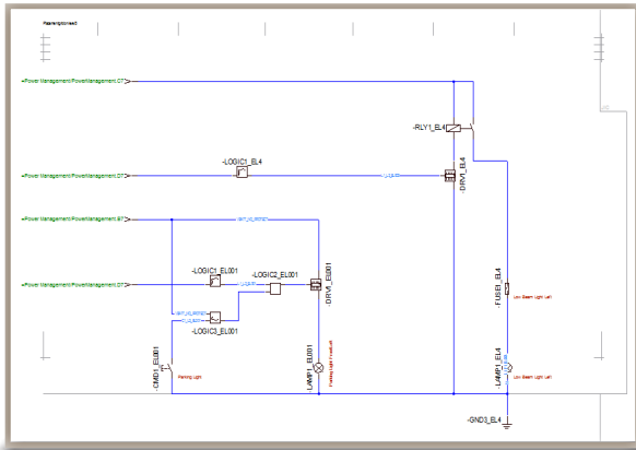
Funktionaler Schaltplan
